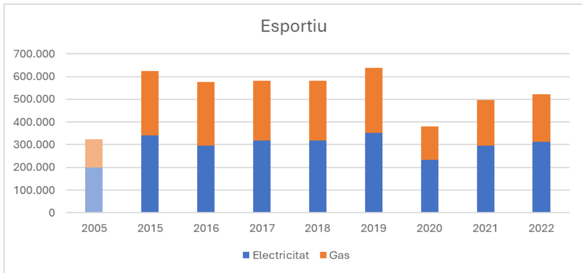
Gràfic 5: Consum energètic anual (kWh) per fonts d'energia dels equipaments esportius. Anys 2005, i 2015-2022.
