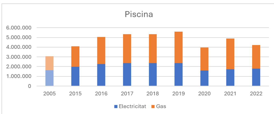
Gràfic 1: Consum energètic anual (kWh) per fonts d'energia dels equipaments amb Piscina. Anys 2005, i 2015-2022.
